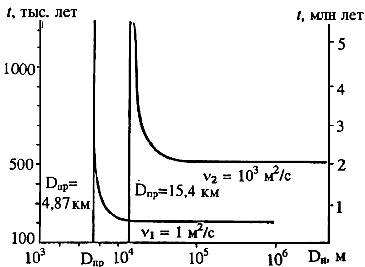
Рис. 4.31. Время выплавления плюма (проплавления канала) в зависимости от диаметра источника для двух разных вязкостей \nu_1 и \nu_2 .
