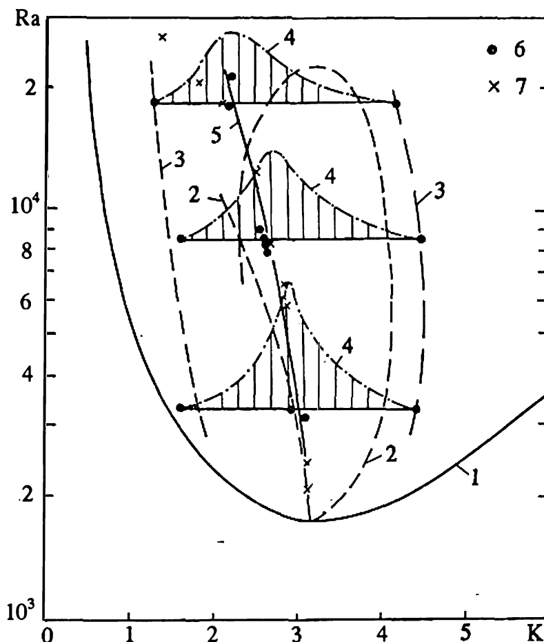
Рис. 3.2. Диаграмма устойчивости конвективных валиков:
