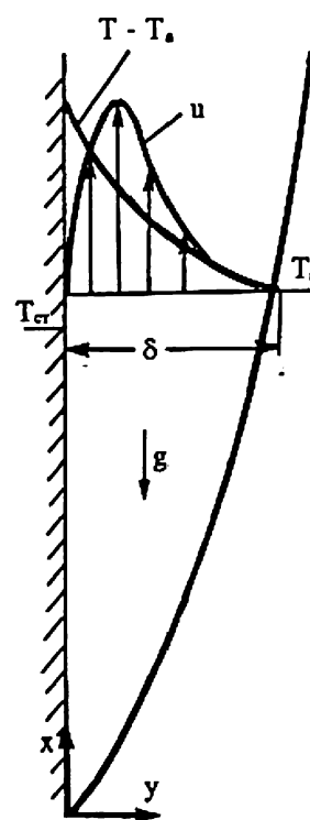
Рис. 2.13. Пограничный слой у вертикальной плоской пластины при тепловой гравитационной конвекции.
