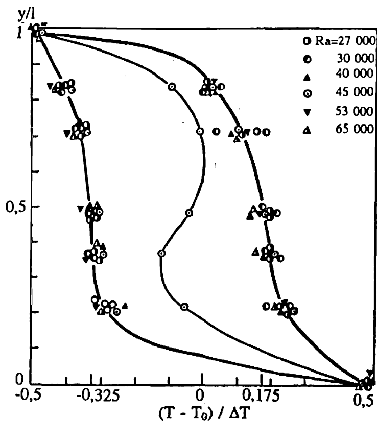
Рис. 3.8. Профили относительной температуры в опускном и подъемном потоках полигональной ячейки по высоте слоя жидкости [Кирдяшкин, 1966].
