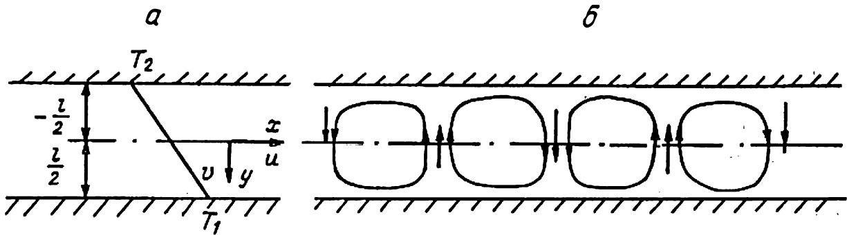
Рис. 3.1. Схема течения жидкости в горизонтальном слое.
