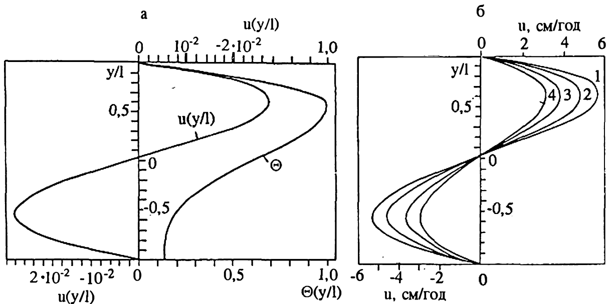
Рис. 5.22. а – профили скорости ( u ) и приведенной температуры ( \Theta ) в горизонтальном слое при локальном подводе тепла и охлаждения сверху; б – профили скорости в астеносфере при Q = 187,7 кВт/м; x_o = 2732 км; \nu = 2,2 \cdot 10^{15} м 2 /с; x_1/l = 46,1 ; 2l = 250 км.
