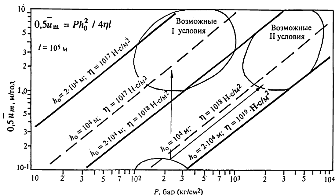
Рис. 5.57. Средняя скорость течения в аккреционном клине в зависимости от средней величины внешнего давления ( P ), вязкости ( \eta ) и высоты клина ( h_0 ).
