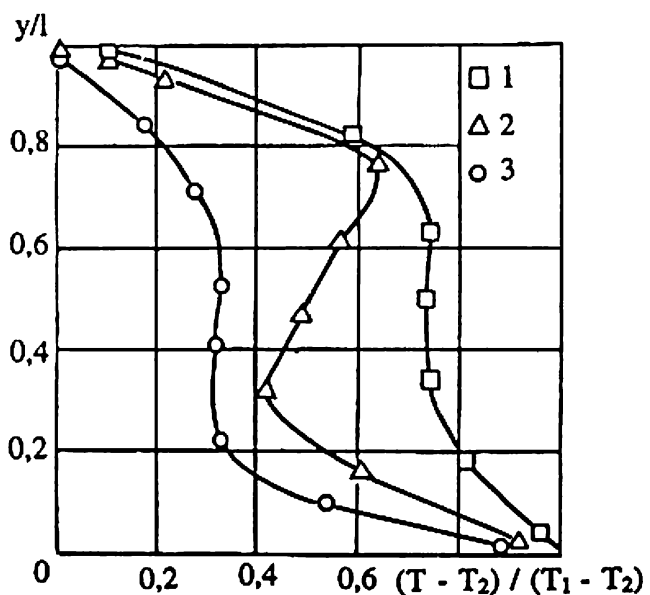
Рис. 3.6. Профили температуры в валике [Бердников, Кирдяшкин, 1978]:
