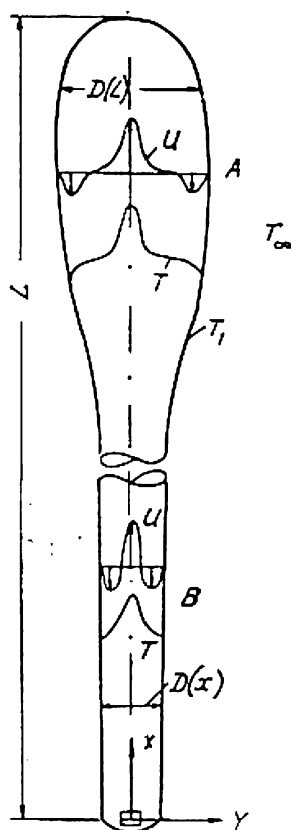
Рис. 4.23. Схема режимов свободно-конвективных течений в расплаве: А – режим пограничного слоя; В – режим теплопроводности.
