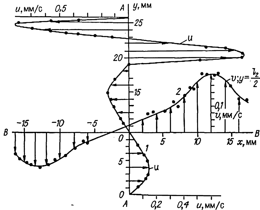
Рис. 4.8. Профили скорости в горизонтальной двухслойной системе жидкостей: глицерин (нижний слой) и гексакан (верхний слой). Составляющие скорости: u – горизонтальная, v – вертикальная; оси x , y и положение сечений A – A и B – B показаны на рис.4.7.
