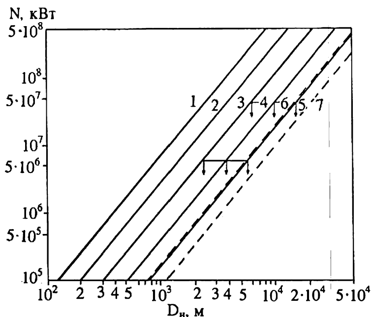
Рис. 4.28. Зависимость мощности источника тепла от его размера D_n и перепада температуры \Delta T_o = T_o - T_n при \lambda_{ж} = 4 \text{ Вт/м}^\circ\text{С} по соотношению (4.20):
