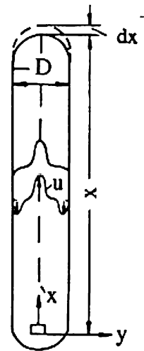
Рис. 4.29. Схема нестационарного выплавления канала над локальным источником тепла.
