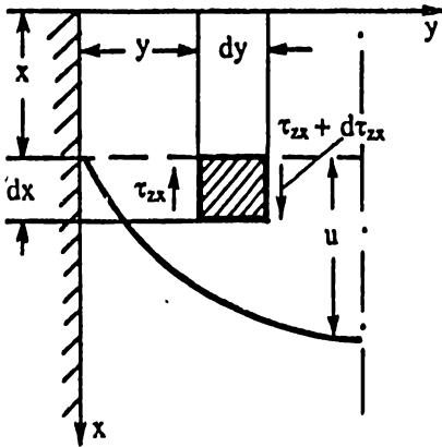
Рис. 2.12. Направления касательных напряжений, действующих на элемент жидкости в одномерном потоке.
