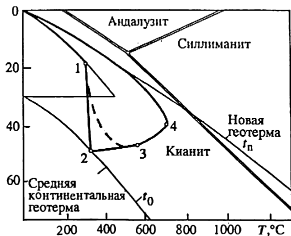
Рис. 5.62. Эволюция P - T -условий в ходе утолщений континентальной коры и коллизионного метаморфизма [England, Thompson, 1984]:
