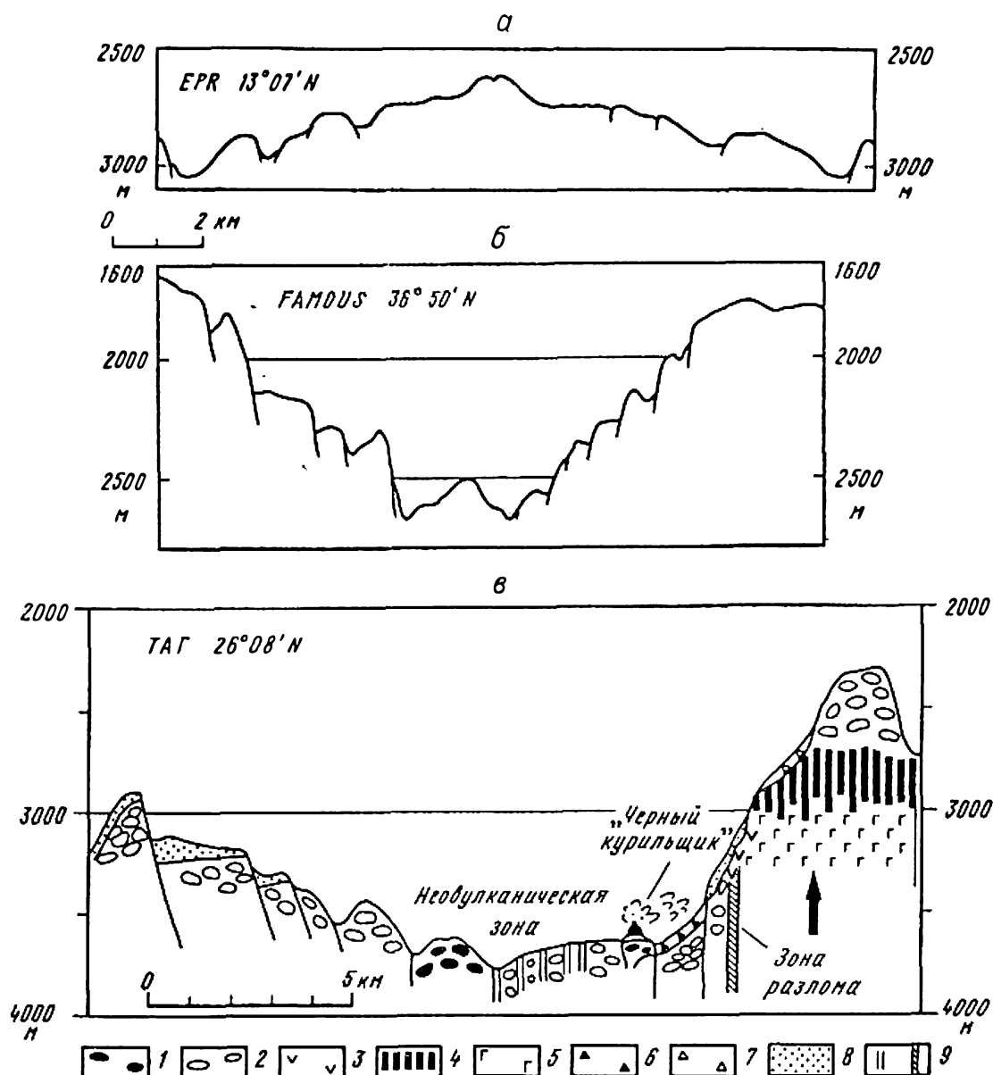
Рис. 5.7. Разрезы осевой части СОХ – быстроспредингового Восточно-Тихоокеанского поднятия (а) и медленноспредингового Срединно-Атлантического хребта – в районе FAMOUS (б) и в районе ТАГ, геологический разрез (в).
