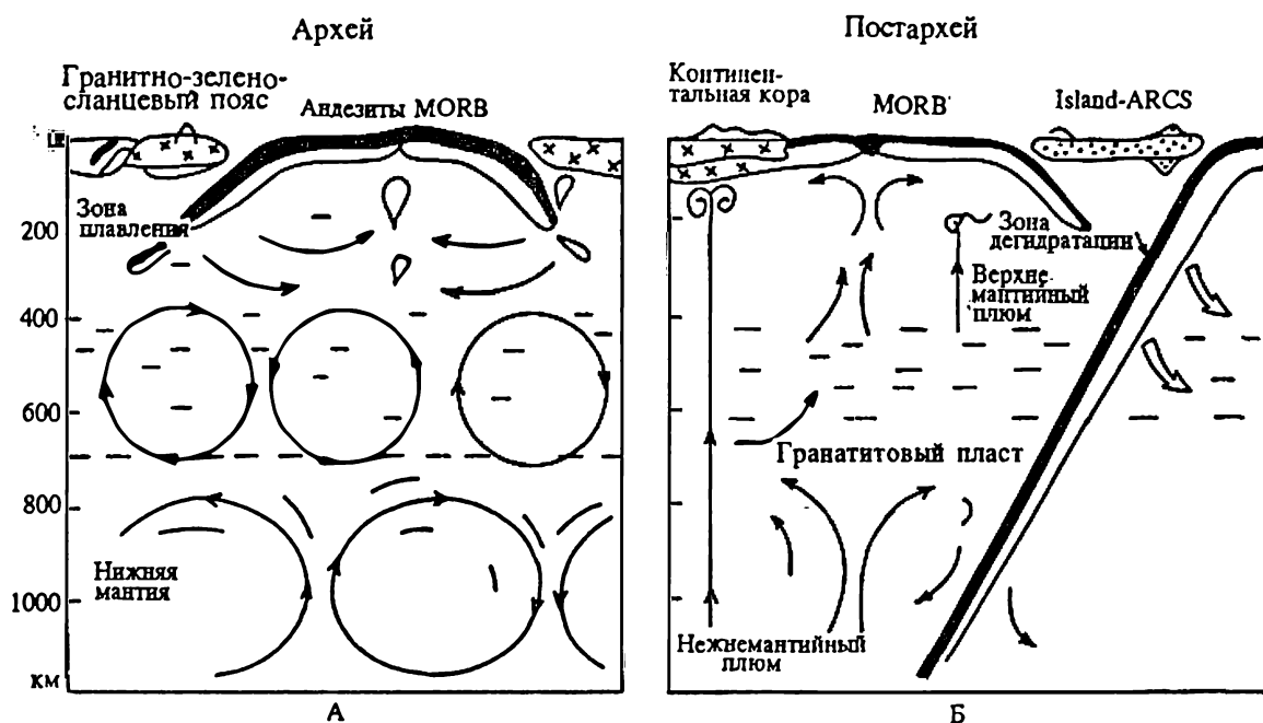
Рис. 4.20. Схема, иллюстрирующая режимы архейской и постархейской мантийной конвекции [McCulloch, 1993]; ограниченная (до 200 км) субдукция и трехслойная конвекция характерны в архее (А); в постархейское время картина субдукции и конвекции ближе к современной (Б).
