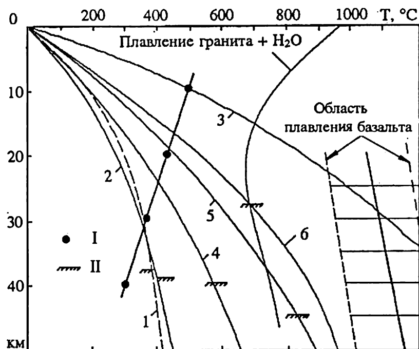
Рис. 2.9. Распределение температуры по глубине для Сибири и Камчатки. Пояснения см. в табл. 2.3: I – температура Кюри титаномагнетитов в зависимости от глубины их формирования; II – положение границы “М”.
