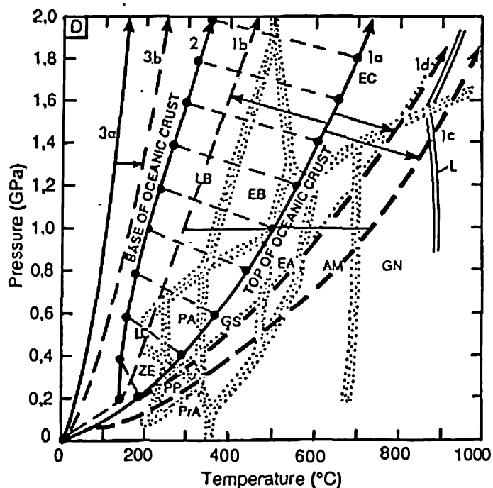
Рис. 5.49. Рассчитанные распределения T и P в модели [Реасоск, 1993] на фоне схемы метаморфических фаций. Фации: ZE – цеолитовая, PP – пре-нит-пумпеллиитовая, PrA – пре-нит-актинолитовая, LC – лавсонит-хлоритовая, PA – пумпеллиит-актинолитовая, GS – зелено-сланцевая, EA – эпидот-амфиболитовая, AM – амфиболитовая, GN – гранулитовая, LB – лавсонит-голубосланцевая, EB – эпидот-глаукофановая, EC – эклогитовая (сравни с рис. 5.48 и 5.51). Линии 1a, 1b, 1c, 1d, 2, 3a, 3b – см. объяснения в тексте, L – линия плавления в присутствии H_2O .
