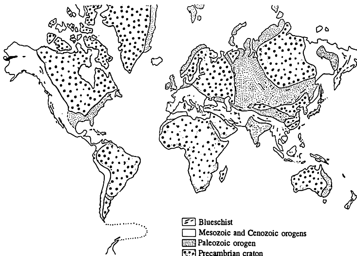
Рис. 1.1. Распространение докембрийских кратонов и фанерозойских орогенических поясов [Магуама, 1994]. Черные штрихи и линзы в складчатых областях - голубые сланды и офнолиты. Палеозойские пояса, сформировавшиеся на ленте палеозойских палеоокеанов, показаны точечным крапом.
