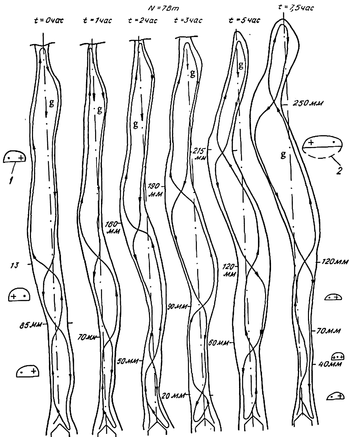
Рис. 4.25. Характер изменения во времени границы раздела расплав – поликристаллический массив (эйказан) при плавлении над локальным источником тепла: D_n = 15 мм, N = 7 Вт и T_{\text{ст}} = 21 °С; 1 – поперечное сечение канала для различной высоты ( x ); g – ускорение силы тяжести. Остальные пояснения см. в тексте.
