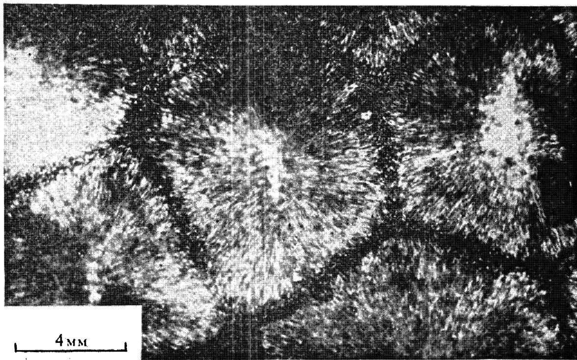
Рис. 3.4. Полигональная форма течения: Pr = 16 , l = 4 мм, Ra = 22\ 600 .
