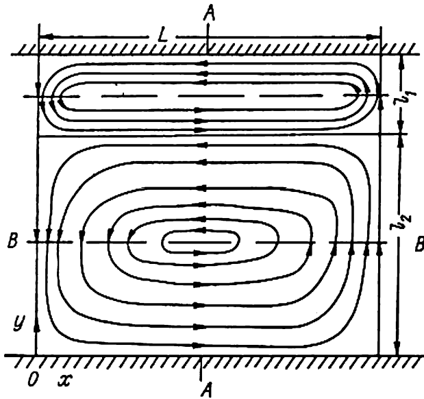
Рис. 4.7. Линии тока в двухслойной системе жидкостей гексадекан–глицерин, определенные из телефильма. В сечениях А – А и В – В определены профили скорости, представленные на рис.4.8.
