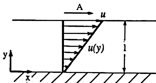
Рис. 2.2. Распределение скоростей в потоке вязкой жидкости между двумя параллельными плоскими стенками (течение Куэтта).
