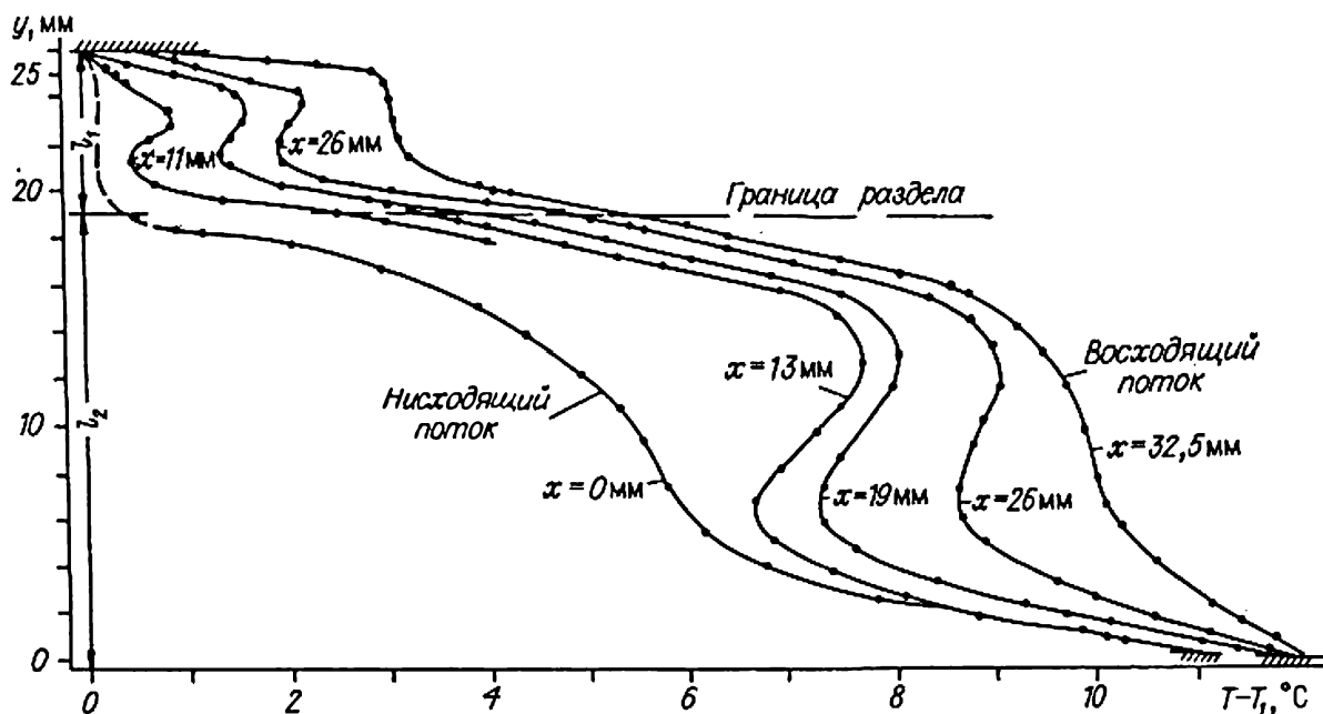
Рис. 4.9. Профили температуры в горизонтальном слое глицерин-гексадекан, определенные в различных вертикальных сечениях от нисходящего течения ( x = 0 ) до восходящего ( x = 32,5 ).
