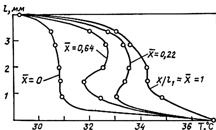
Рис. 3.7. Профили температуры в полигональной ячейке [Кирдяшкин, 1966].
