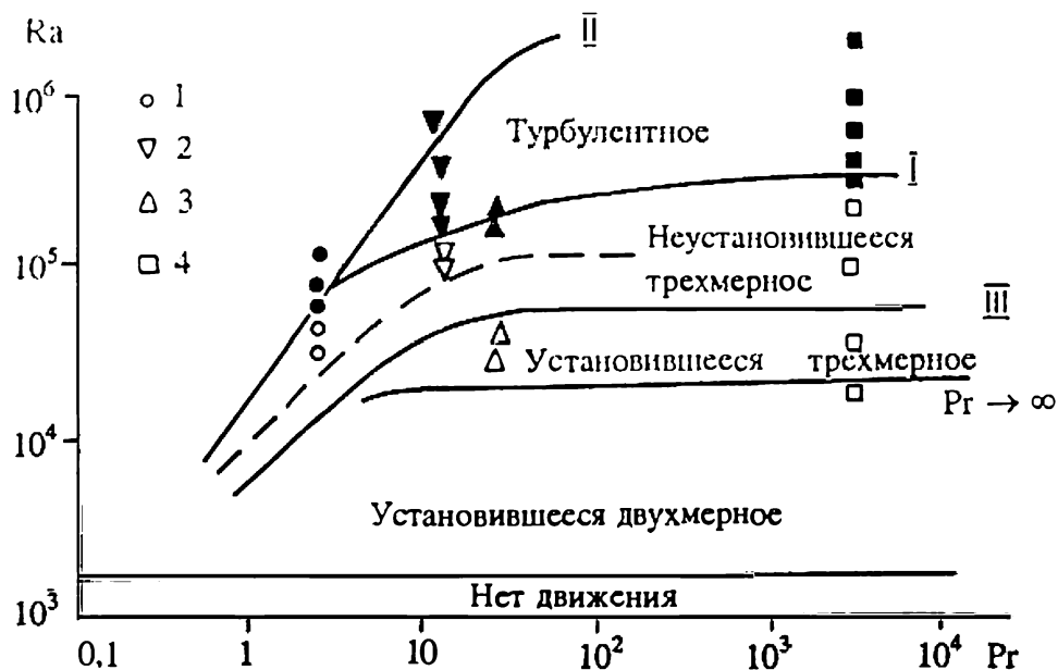
Рис. 3.5. Границы режимов течения.
