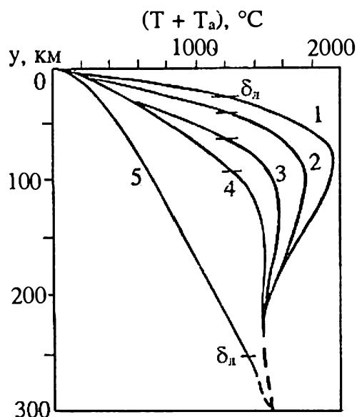
Рис. 5.25. Распределение температуры в астеносфере и литосфере океана (1–3) и континента (4,5) (см. рис.5.24) при x , равном (в км): 1 – 200, 2 – 1000, 3 – 2000, 4 – 3100, 5 – > 4140.
