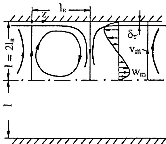
Рис. 5.26. Схема валиковых течений вблизи охлаждающей верхней поверхности.
