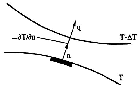
Рис. 2.3. Изотермические поверхности и температурный градиент.
