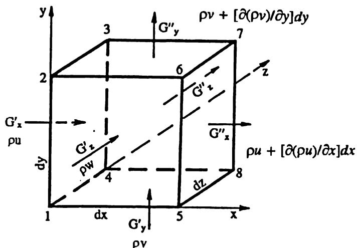
Рис. 2.10. К выводу дифференциального уравнения сплошности.
