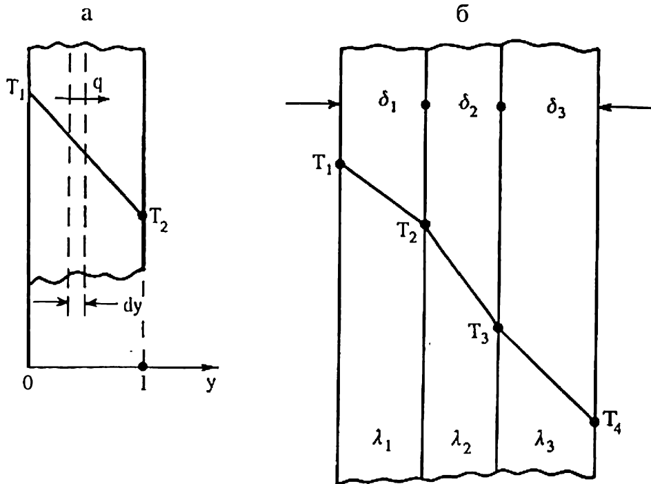
Рис. 2.4. Однородная плоская (а) и многослойная плоская (б) стенки.
