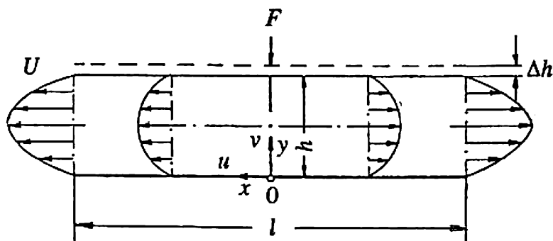
Рис. 5.56. Схема течения вязкой жидкости между сдвигаемыми жесткими пластинами.
