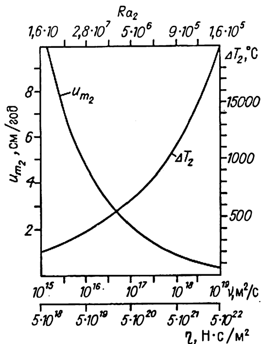
Рис. 4.13. Перепад температуры \Delta T_2 и максимальное значение горизонтальной скорости u_{m2} в нижней мантии, вычисленные по зависимостям (4.10) – (4.12) для различных вязкостей ( \nu и \eta ) и чисел Рэлея ( Ra_2 )
