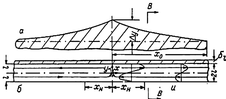
Рис. 5.15. а – схема рельефа СОХ и б – схема движения в астеносфере под СОХ (увеличена по y ).
