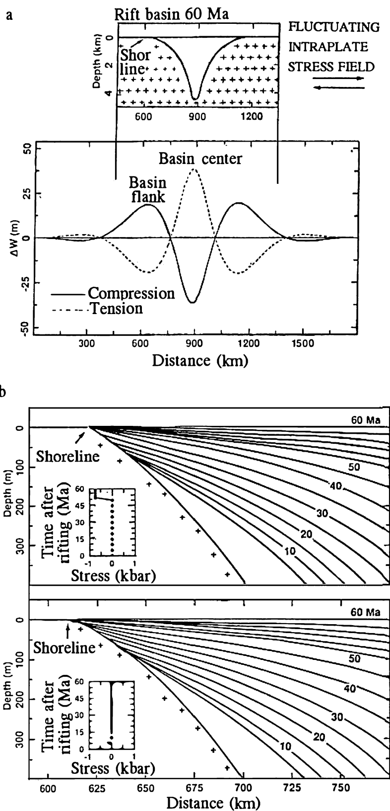
Рис. 5.36. Индуцированные стрессом погружения (поднятия) в рифтовых бассейнах [Cloetingh et al., 1985]:
