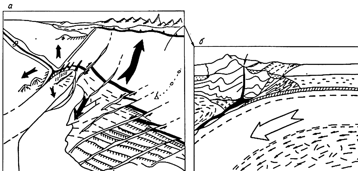
Рис. 1.12. Идеализированные схемы, иллюстрирующие тектонику плит: а – границы расхождения плит в рифтах и океане (зонах спрединга), с трансформными разломами; б – разрез зоны субдукции; заштрихована океаническая кора и выше нее – деформированные породы аккреционной призмы и островной дуги; черное – расплав в зоне субдукции и вулканических аппаратах.
