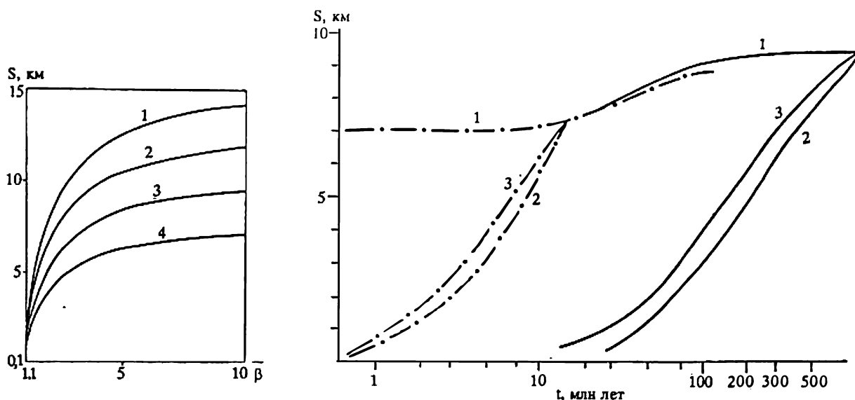
Рис. 5.33. Рассчитанные кривые мощности осадков ( S ) в зависимости от показателя растяжения \beta [Ревердатто и др., 1995]. Цифры 1, 2, 3 и 4 соответствуют мощностям земной коры 30, 40, 50 и 60 км соответственно. Мощность литосферы 125 км.
