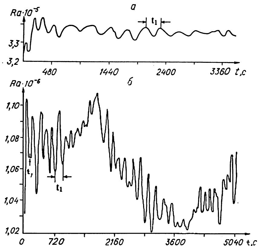
Рис. 3.14. Изменение числа Ra в горизонтальном слое во времени:
