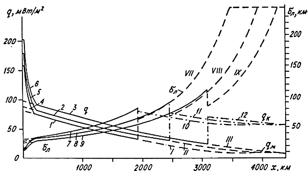
Рис. 5.23. Тепловые потоки и толщина литосферы океана и континента при l = 125 км. Тепловые потоки и литосфера океана по формуле (5.11):
