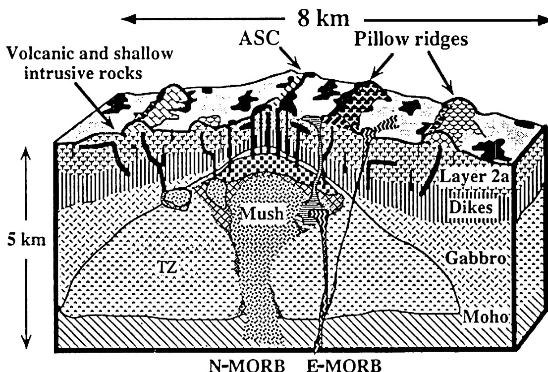
Рис. 5.4. Строение океанической коры участка 9°31' (см. рис. 5.3) с учетом модели магматической камеры, представленной в работе J. Sinton, R. Detrick [1992]. Показано сложное и асимметричное распределение лав, даек и силлов вне осевой кальдеры (ASC). Часть лав происходит из промежуточной зоны (TZ) или в результате смешения с глубинными расплавами типа E-MORB [Perfit et al., 1994].
