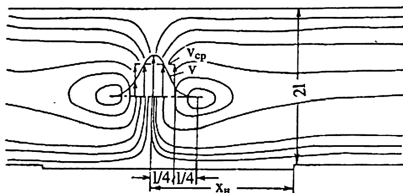
Рис. 5.20. Экспериментальные линии тока в слое глицерина ( 2l = 19 мм; x_H = 1,4l ; Q = 190 Вт/м). Представлен также профиль вертикальной скорости v и принятой в расчете средней скорости v_{ср} .
