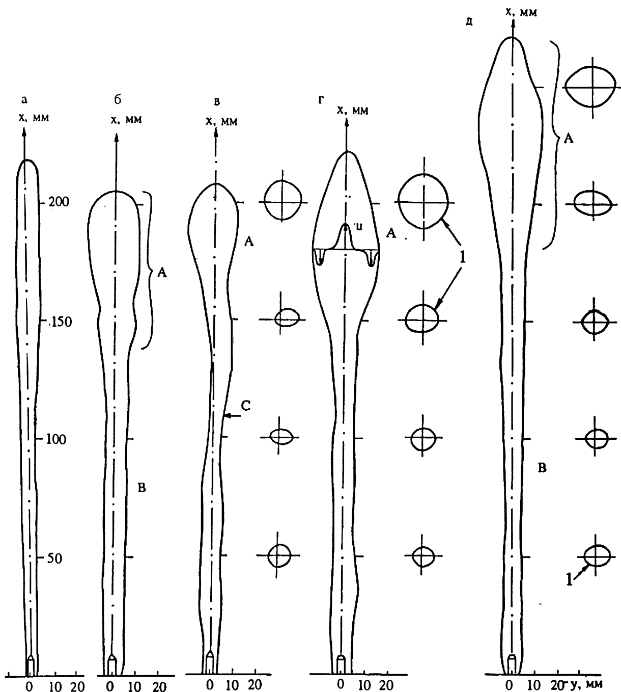
Рис.4.24. Граница раздела расплав – поликристаллический массив парафина при плавлении над локальным источником тепла D_H = 4 мм, когда все тепло отводится в объем парафина.
