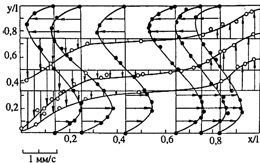
Рис. 3.11. Поле скорости в ячейке полигональной формы:
