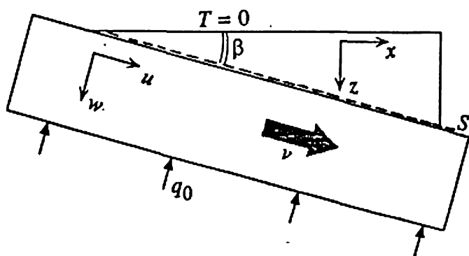
Рис. 5.50. Система координат и геометрия субдукционной зоны в модели [Реасоск, 1993]. Объяснения см. в тексте.
