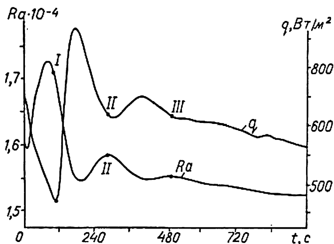
Рис. 3.13. Развитие конвекции в горизонтальном слое глицерина: Pr = 3 \cdot 10^3 ; \overline{Ra} = 1,54 \cdot 10^4 ; l = 17,8 мм.
