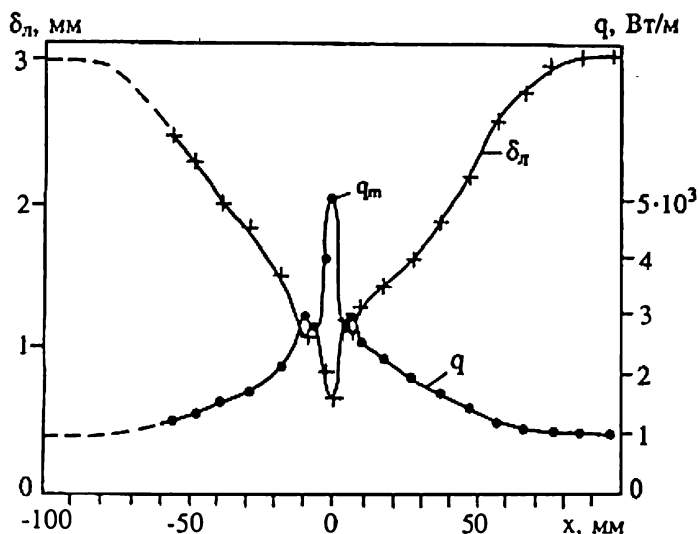
Рис. 5.21. Средние по ширине охлаждающей пластины толщины закристаллизовавшегося октадекана ( \delta_n ) и значения удельных тепловых потоков ( q ) для различных x при 2l = 20 мм; x_n = 0,5l ; T_1 = 19 °С; x_0 = 100 мм.
