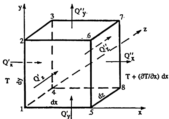
Рис. 2.6. К выводу уравнения теплообмена.
