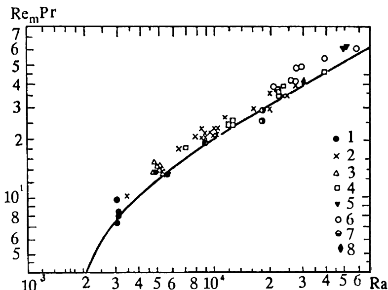
Рис. 3.12. Зависимость Re_m от Ra для Pr \approx 16 по экспериментам В.С. Бердникова и А.Г. Кирдяшкова [1978].
