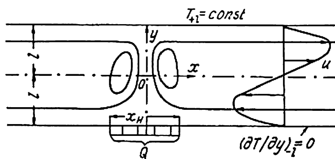
Рис. 5.19. Схема течения жидкости в горизонтальном слое при локальном подводе тепла снизу ( x_H ) и охлаждении сверху.
