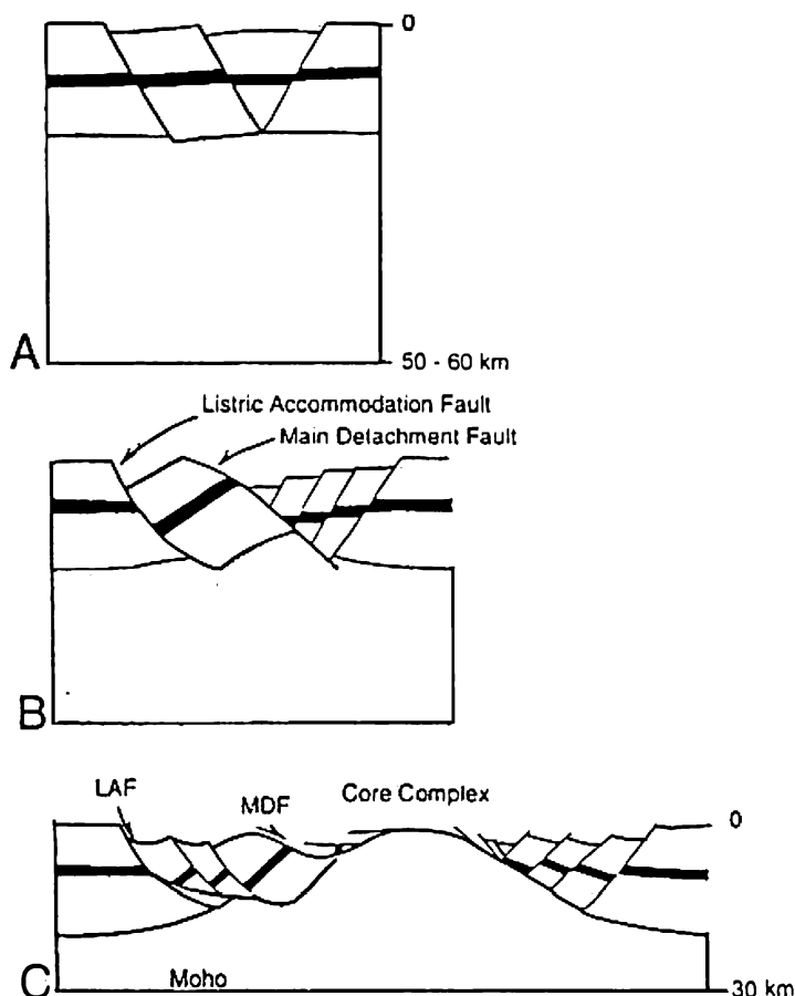
Рис. 5.38. Эволюционная модель системы с разделительным разломом по результатам экспериментального моделирования [Brun et al., 1994].
