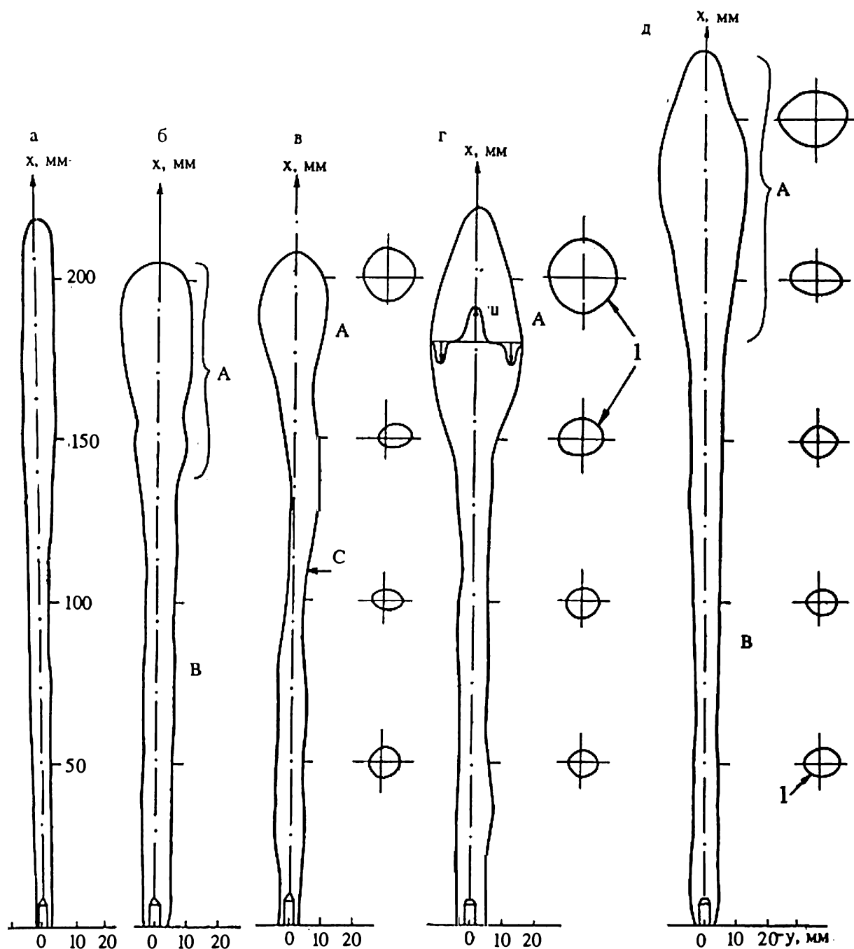
Рис. 4.24. Граница раздела расплав – поликристаллический массив парафина при плавлении над локальным источником тепла D_n = 4 мм, когда все тепло отводится в объем парафина.
