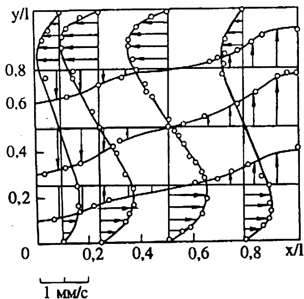
Рис. 3.10. Поле скорости в ячейке валиковой формы:
