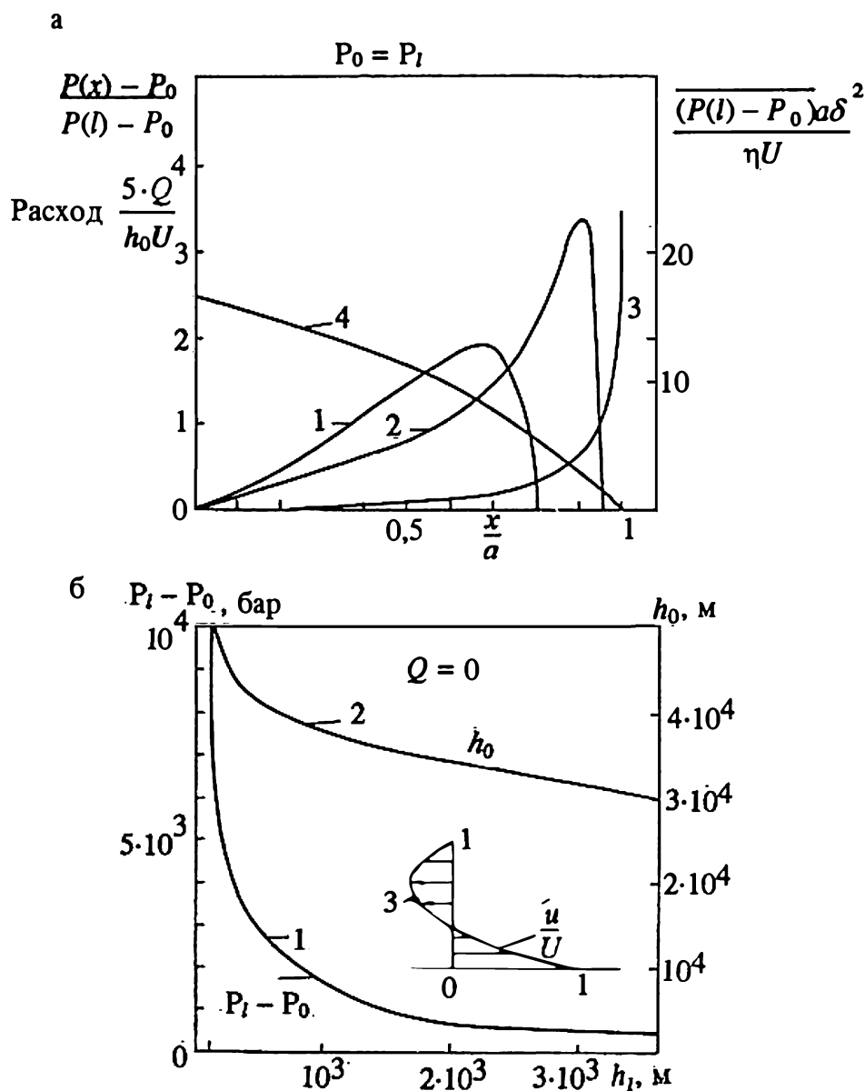
Рис. 5.53. Модель вязкого клина между взаимодействующими плитами:
