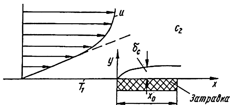
Рис. 3.17. Схема массопереноса в концентрационном - пограничном слое.
